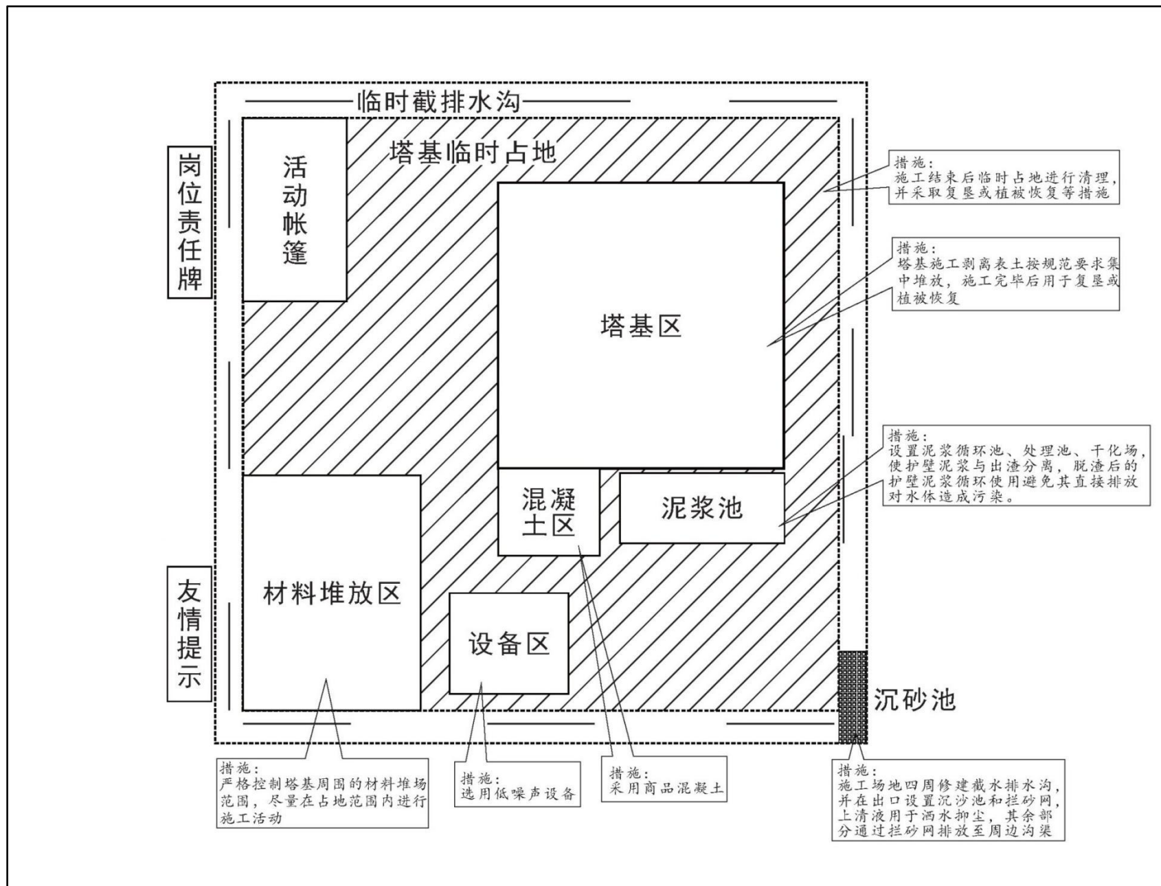
附图 6 本项目输电线路塔基环境保护措施布置图
