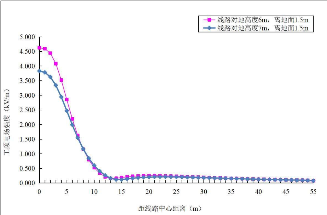
图 3-2 110-EC21GS 型塔（同相序）工频电场强度随距原点距离变化曲线
