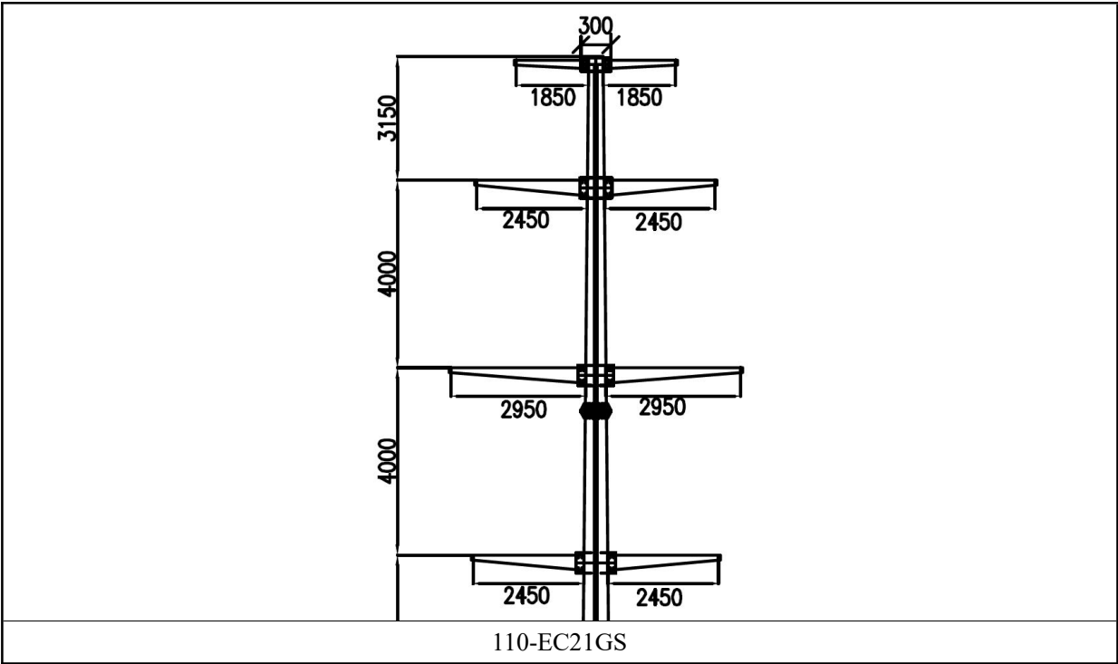
图 3-1 预测塔型图
