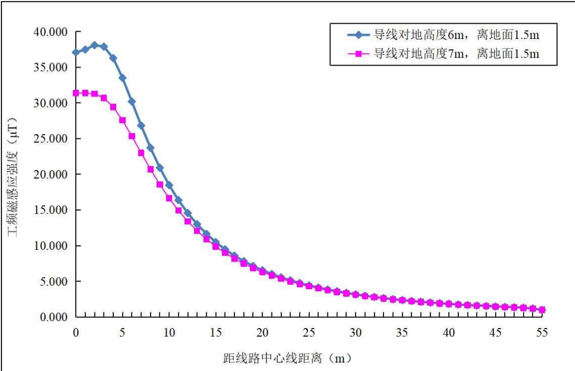
图 3-3 110-EC21GS 型塔（同相序）工频磁感应强度随距原点距离变化曲线
