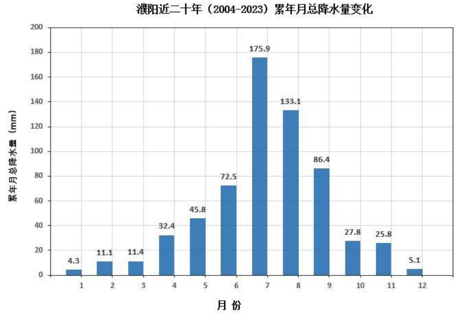
图 4-5 濮阳（2004-2023）月平均降水量（单位：毫米）
