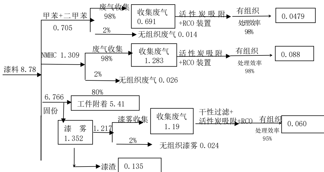
图2-1 本项目漆料平衡图 (t/a)
